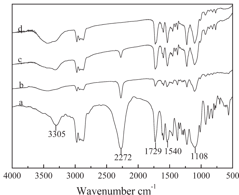
Figure 2 FTIR spectra of the PU: (a) 3 min, (b) 2 h, (c) 4 h, and (d) 5 h.
